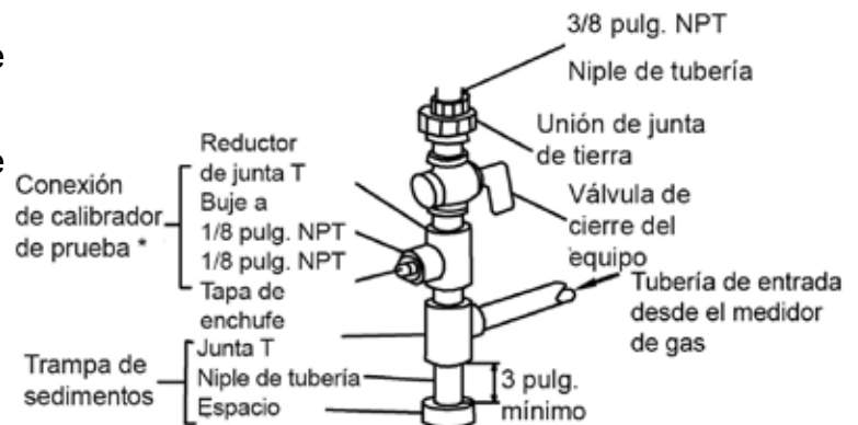
Fig. 17 - Conexión del gas
