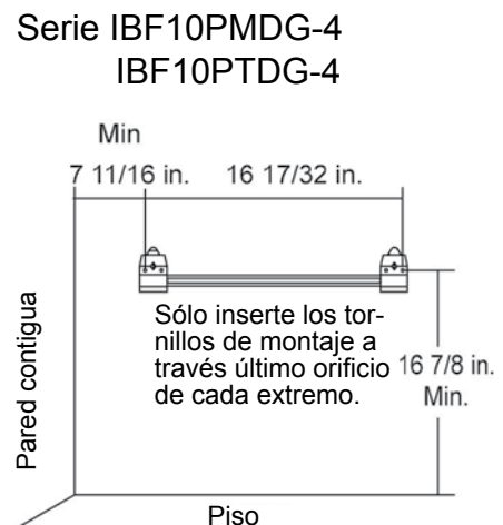
Fig. 13 - Soporte de montaje Separadores (pulgadas)
