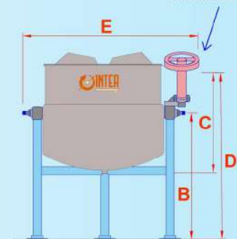
Mecanismo de volteo: Tornillo Sinfin
