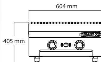
FRONTAL
