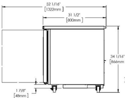
VISTA LATERAL
