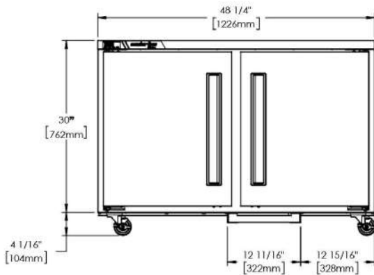
ELEVACIÓN
