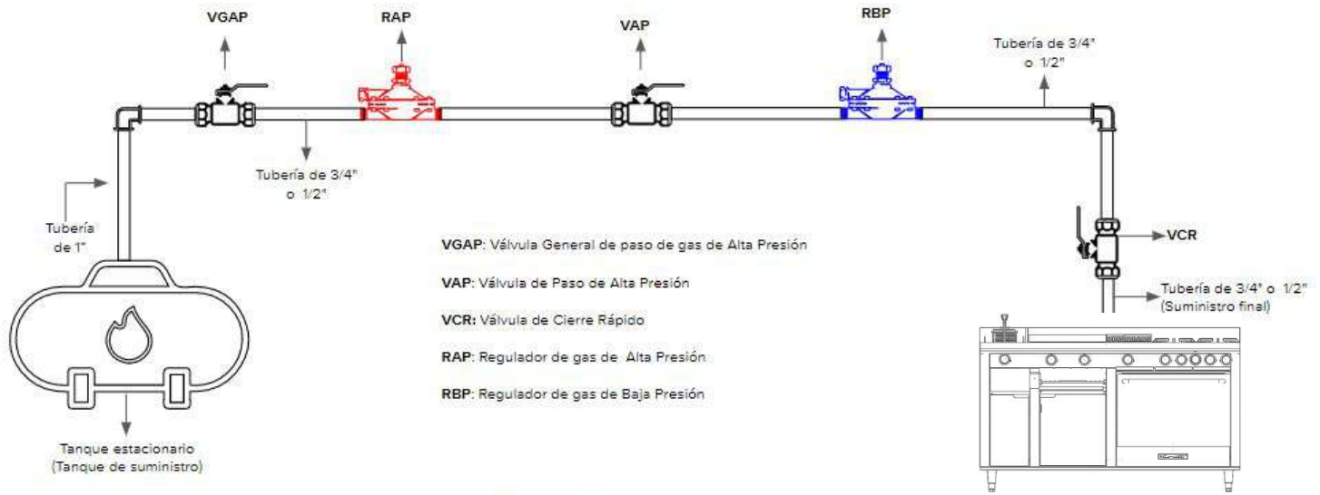
Diagrama 1. Instalación de gas para 1 equipo
