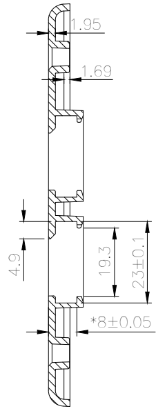
Profile A-A
