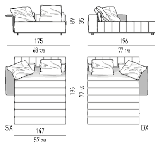
CHAISE-LONGUE CM 175X196
