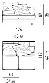
ELEMENTO CENTRALE CM 126 CENTRAL ELEMENT CM 126
