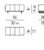
GRAY TAVOLINO | COFFEE TABLE
