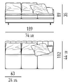
ELEMENTO CENTRALE CM 189 CENTRAL ELEMENT CM 189
