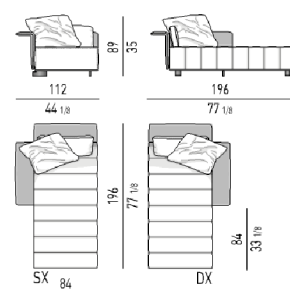
CHAISE-LONGUE CM 112X196
