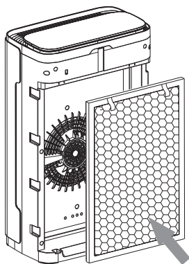
4. 裝入納米礦晶過濾器
