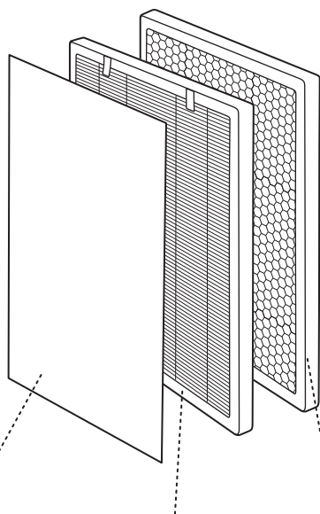
初效濾網 高效銀離子空氣過濾器 納米礦晶過濾器
