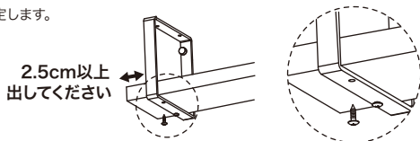
3段棚
