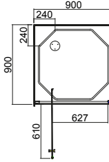
900 x 900 FLAT WALL IPAIW999FL9C
