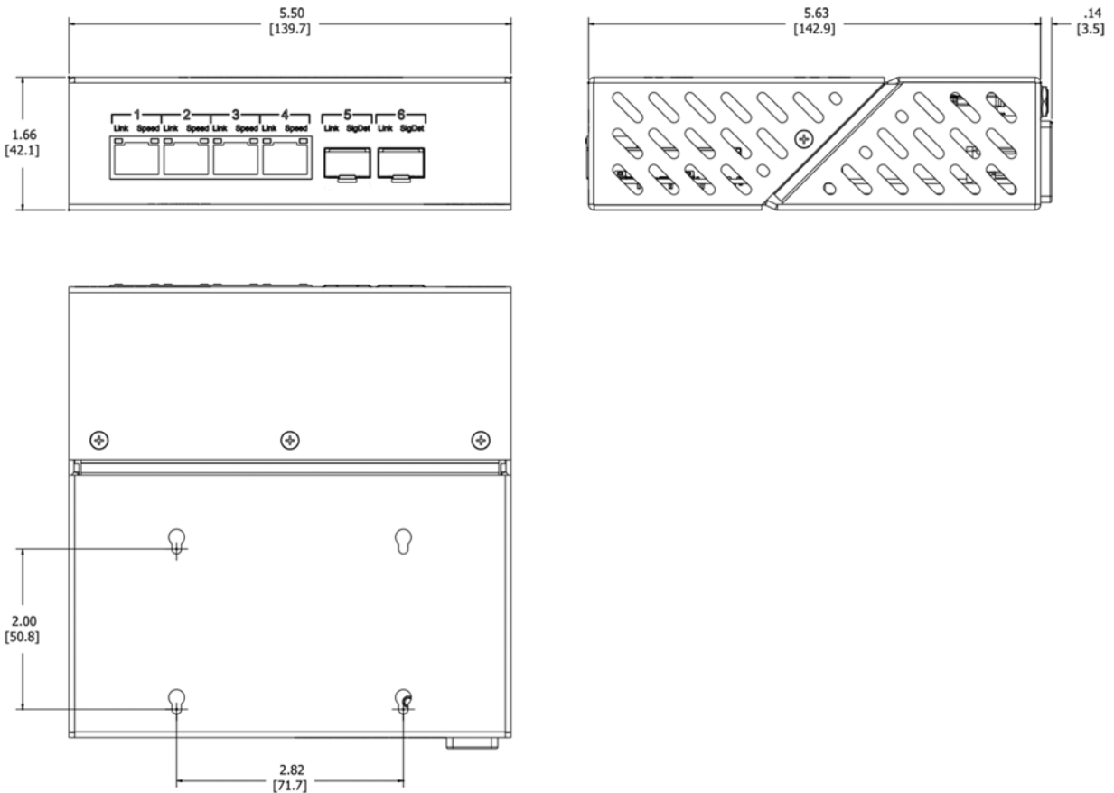
Figure 18. FP1004E Dimensions
