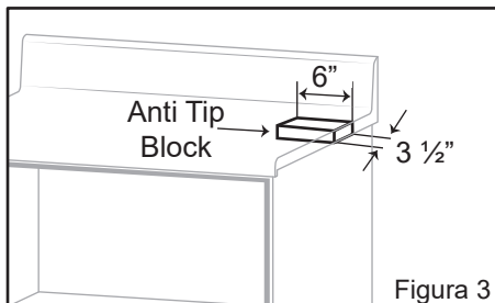
BLOQUE ANTI-TIP
