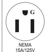
NEMA 5-15P
