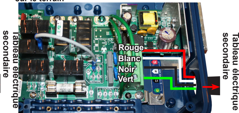
Boîtier de contrôle de 110/230 volts pour conversion sur le terrain
