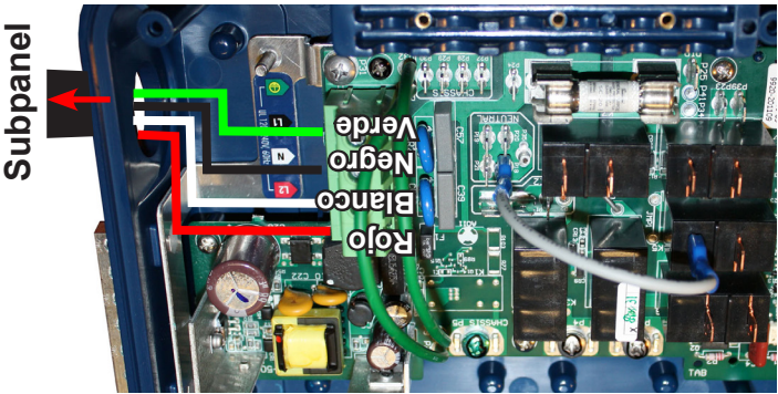
Caja de control de campo de conversión 110 V 30 A
