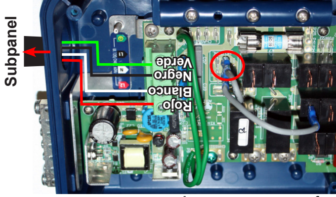
Caja de control de campo de conversión 110/230 V
