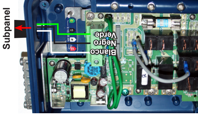
Caja de control de campo de conversión 110 V 30 A
