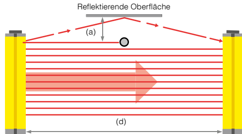
ABB. 11: ABSTAND ZWISCHEN REFLEKTIERENDER OBERFLÄCHE UND SCHUTZFELD ZU KLEIN; EIN REFLEKTIERTER LICHTSTRAHL TRIFFT UNABSICHTLICH AUF DEN EMPFÄNGER
