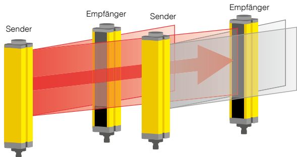
ABB. 14: STÖRUNG ZWISCHEN ZWEI BWS-PAAREN
