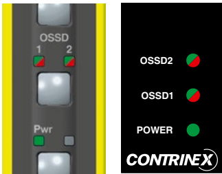
ABB. 8B: LED-ANZEIGE EMPFANGSEINHEIT
