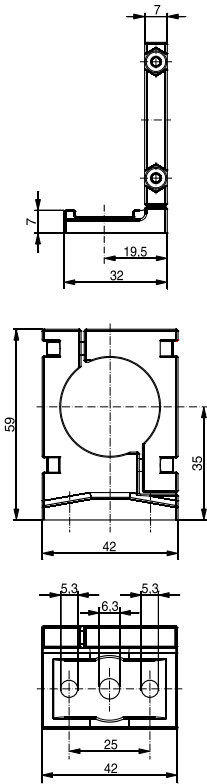
ABB. 17: MONTAGEHALTERUNG (BEZ. YXW-0001-000)
