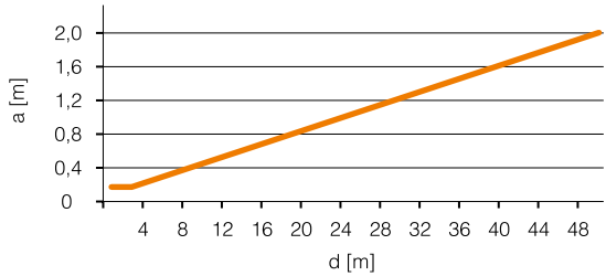
DIAGRAMM 4: ABSTAND ZWISCHEN STRAHLEN UND REFLEKTIERENDER OBERFLÄCHE (a) HÄNGT VOM ERFASSUNGSBEREICH (d) AB
