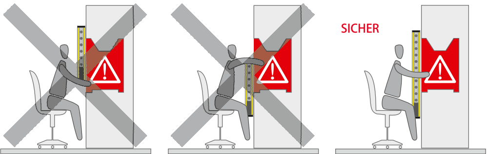
ABB. 4: ANORDNUNG DES LICHTVORHANGS
