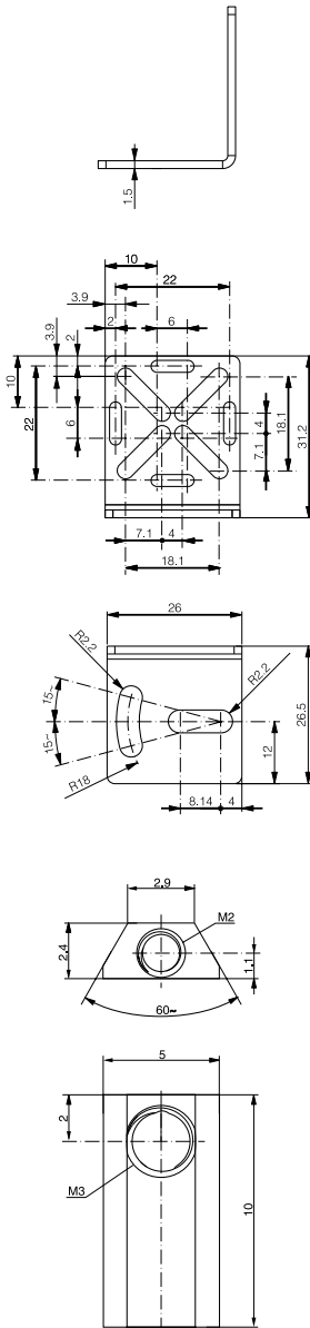
ABB. 23.1: SONDERHALTERUNG FÜR GERÄTEENDEN NR. 7 (REF: YXW-0007-000)
