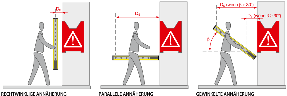
ABB. 6: MINDESTSICHERHEITSABSTAND (U.S. UND KANADA)
