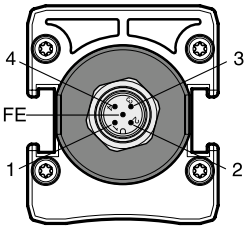
ABB. 24: M12-ANSCHLUSSBELEGUNG
