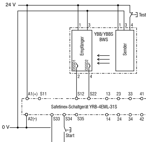
ABB. 29: ANSCHLUSSSCHEMA FÜR HANDSTART-MODUS
