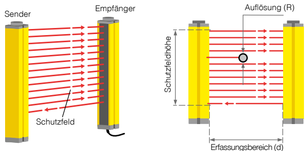
ABB. 2: FUNKTIONSPRINZIP
