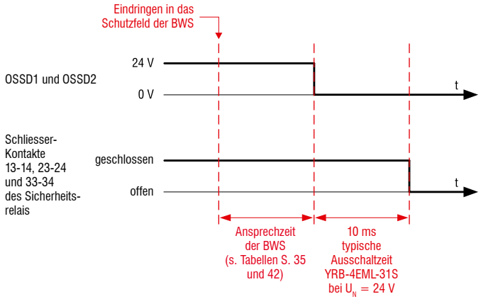
ABB. 28: SCHALTABLAUF DES SICHERHEITSRELAIS
