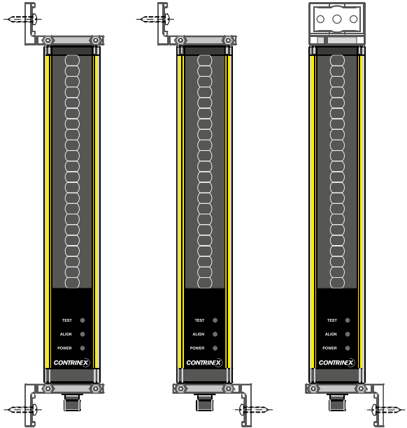
ABB. 18: BEFESTIGUNGSMÖGLICHKEITEN MIT MONTAGEHALTERUNG
