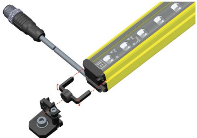
ABB. 21.1: STANDARDHALTERUNG FÜR GERÄTEENDEN NR. 5 (REF: YXW-0005-000)
