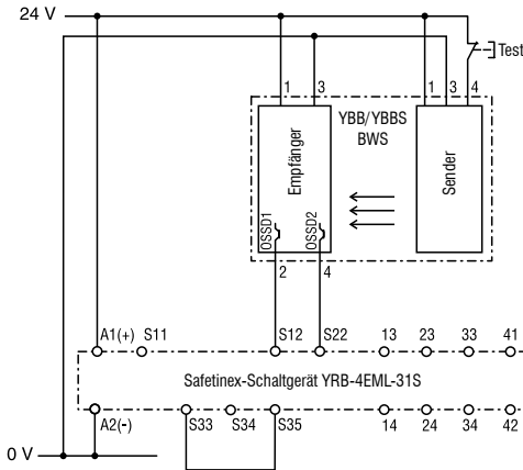
ABB. 30: ANSCHLUSSSCHEMA FÜR MODUS «AUTOMATISCHER START»
