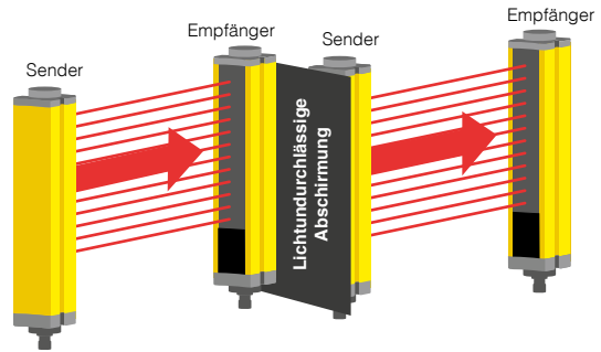
ABB. 15: LICHTUNDURCHLÄSSIGE ABSCHIRMUNG ZWISCHEN ZWEI BWS-PAAREN
