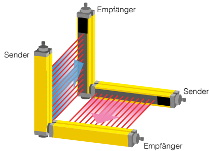
ABB. 16: L-FÖRMIGE INSTALLATION: ENTGEGENLAUFENDE STRAHLEN-RICHTUNG
