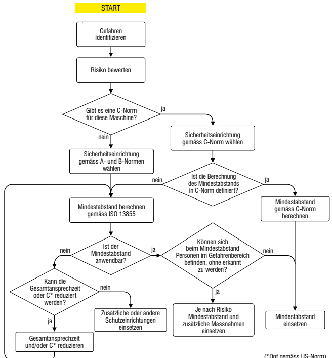
DIAGRAMM 3: BESTIMMUNG DES MINDESTSICHERHEITSABSTANDS
