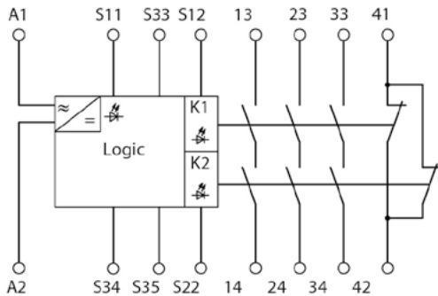
ABB. 27: RELAIS-BLOCKSCHALTBIKD
