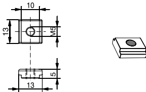
ABB. 19: BEFESTIGUNGSMUTTER (BEZ. YXW-0003-000)
