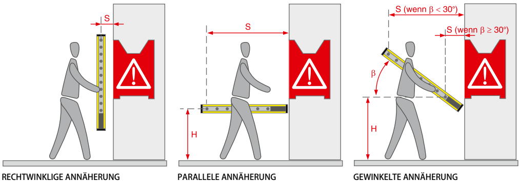
ABB. 5: MINIMUM SICHERHEITSABSTAND (EU)
