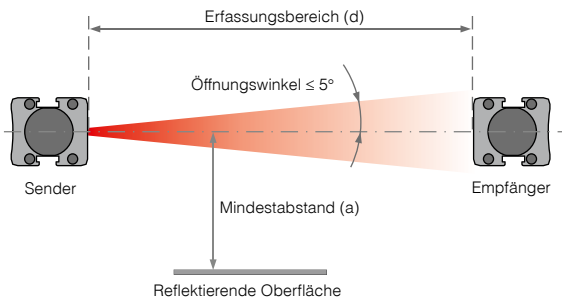
ABB. 12: ABSTAND ZWISCHEN REFLEKTIERENDER OBERFLÄCHE UND SCHUTZFELD IST KORREKT; ES ENTSTEHEN KEINE UNGEWOLLTEN REFLEXIONEN
