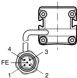
ABB. 25: M12-ANSCHLUSSBELEGUNG
