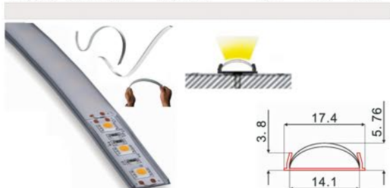
Perfil flexible doblable para realizar formas a medida con tiras LED. Para la iluminación de ventanas, curvas y formas personalizadas.
