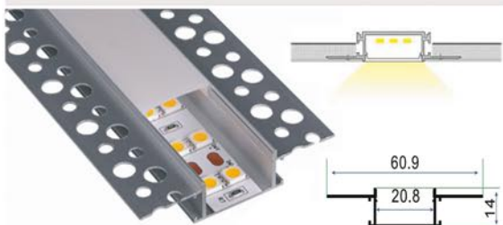
Perfil ancho de pladur para tiras de LED con una iluminación más arquitectural para iluminar utilizando tiras de alta potencia.
