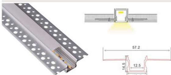
Perfil micro para tiras LED en techos de pladur o escayola, para una iluminación lineal invisible integrada.
