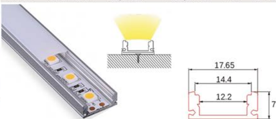
Metro perfil aluminio superficie micro para todo tipo de instalaciones con tiras de LED. En aluminio resistente para una correcta disipación.
