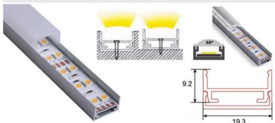
Perfil compuesto por dos partes una guía para canalizar el cable y el aluminio para instalar la tira de LED. Difusor óptico con grados.
