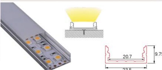
Perfil de aluminio superficie ancho para tiras de LED dobles. Para cualquier instalación, con barra lineal para dos tiras.
