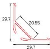
Perfil grande en esquina de 30x30 con difusor redondeado. Para mostradores o luces de alta potencia.
