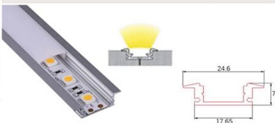
Perfil aluminio de empotrar con aletas micro para integrar en muebles techos y paredes. Perfil micro aletas para tiras de LED flexibles.
