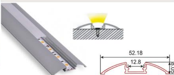
Perfil para realizar contornos de escaleras, suelos o como rodapiés. Para contornos en las zonas para señalizar, no pisable.
