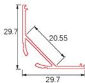
Perfil aluminio grande de esquina con difusor cuadrado 30x30 para instalar doble tira de LED.
