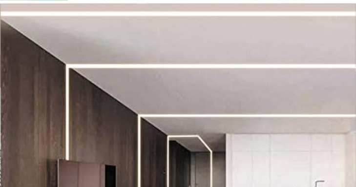
Perfil ancho de pladur para tiras de LED con una iluminación más arquitectural para iluminar utilizando tiras de alta potencia.
