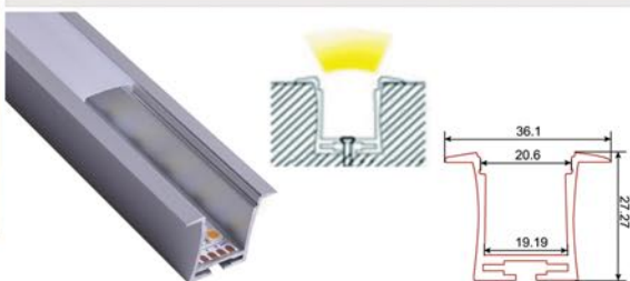
Perfil de aluminio grande para empotrar de 36 x 27cm. Iluminar con tiras de LED de alta potencia en techos.
