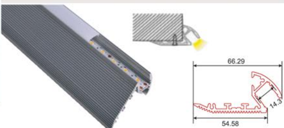
Perfil para iluminar escalones con zona pisable, para dar luz a las escaleras marcando el paso.
