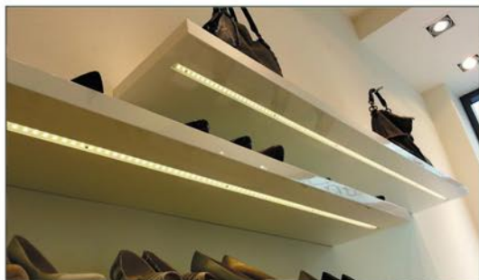
Perfil aluminio de empotrar con aletas micro para integrar en muebles techos y paredes. Perfil micro aletas para tiras de LED flexibles.
