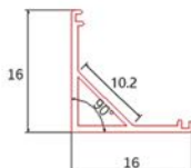
Perfil de esquina 45° con difusor redondeado 16x16. Para instalar tiras de LED de una línea.
