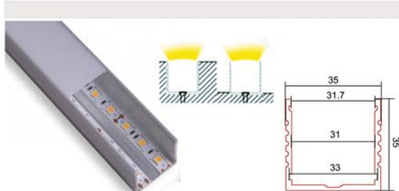
Perfil grande de superficie de 35x35, para tiras de LED de alta potencia. Luz de superficie para realizar luminarias.
