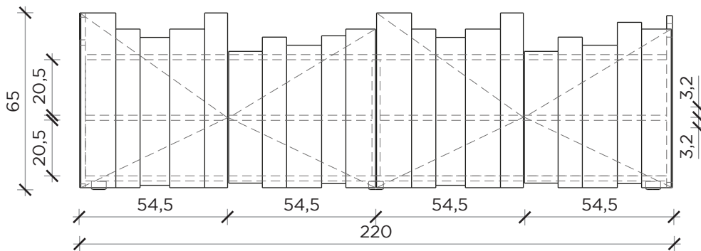
PIANTA | PLAN
