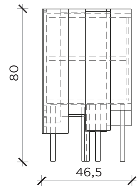
LATO | SIDE
