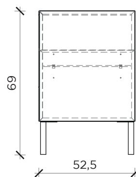
LATO | SIDE
