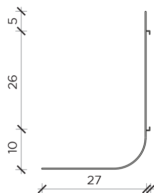
LATO | SIDE
