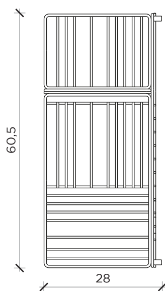
LATO | SIDE
