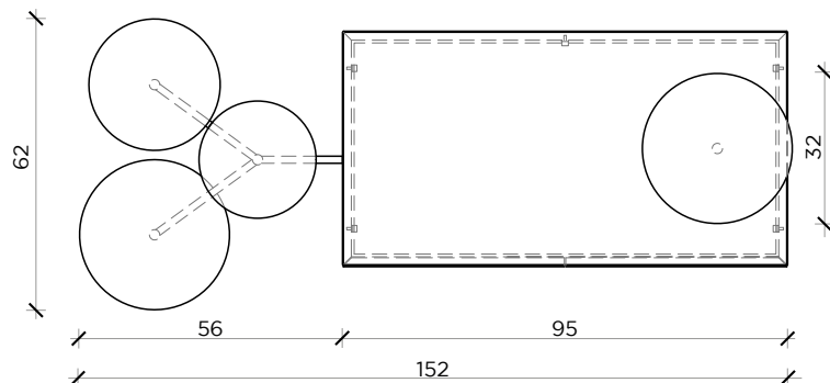
PIANTA | PLAN
