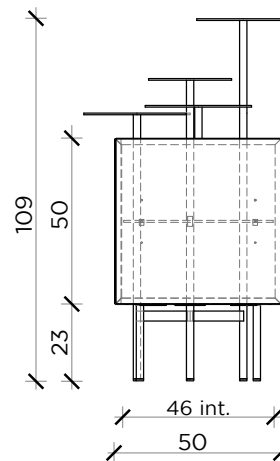
LATO | SIDE
