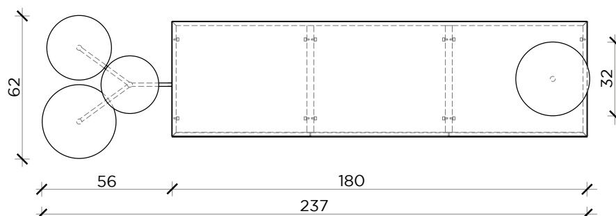
PIANTA | PLAN
