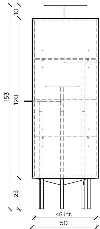
LATO | SIDE
