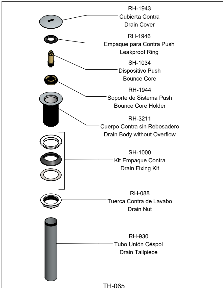
Contra de Push para Lavabo sin Rebosadero Lavatory Push Drain without Overflow
