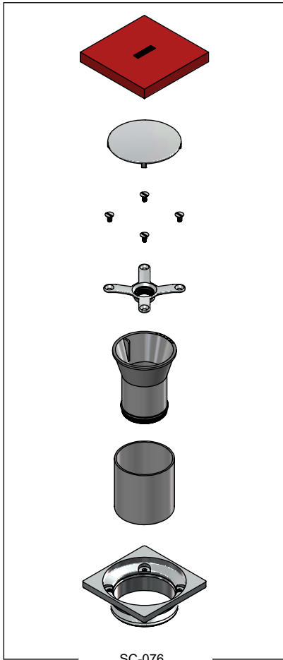
Sub ensamble Contra con Cúpula Floor Drain Strainer Kit
