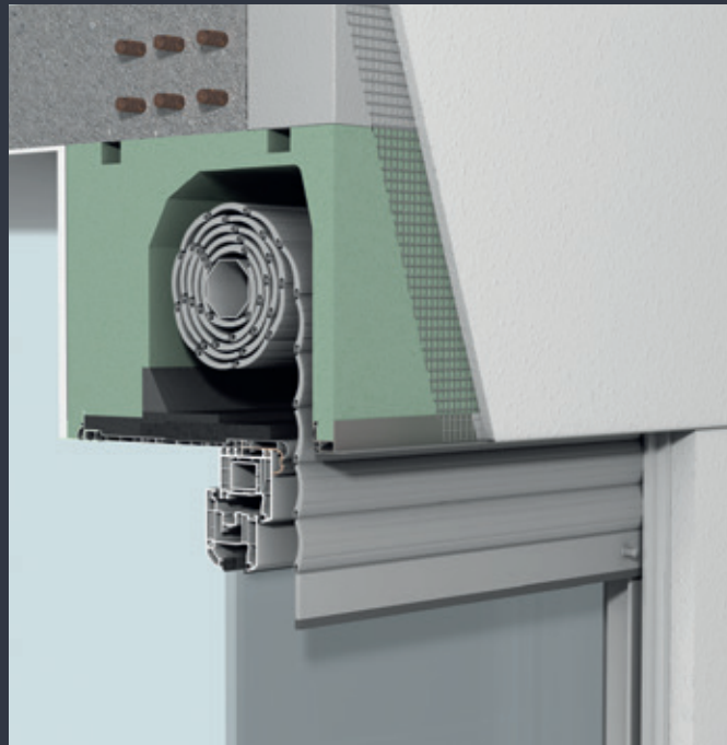
Neubau-Rollladen RollTop II
