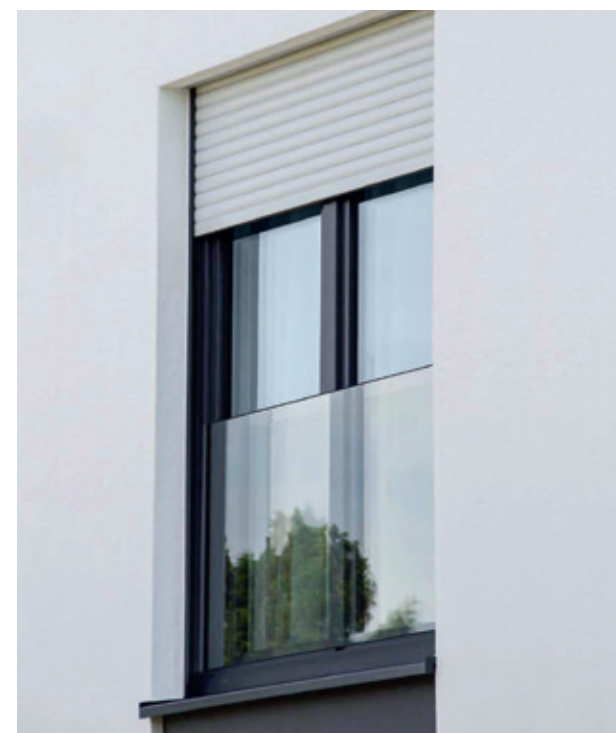
NEXT RG mit Absturzsicherung
