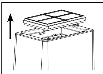
b. Retirez la combinaison de filtres de l'appareil. Remarque : le préfiltre et le filtre au charbon sont combinés en un seul filtre qui s'accroche au filtre HEPA par une bande Velcro.
