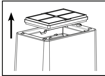
b. Saque el filtro combinado de la unidad. Nota: El prefiltro/filtro de carbón se sujeta al filtro HEPA con una cinta Velcro.
