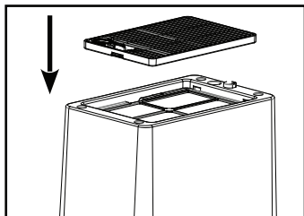
e. Vuelva a colocar la cubierta posterior de la unidad y asegúrela en su sitio.
