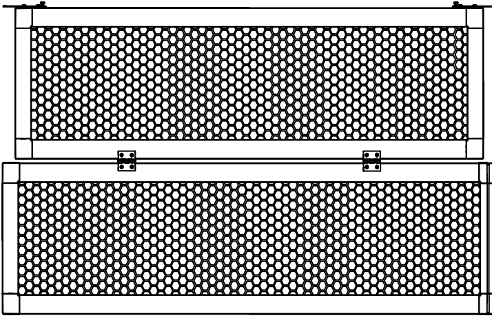
11174 FENCE PANEL B - PANNEAU DE CLÔTURE B - PANEL DE VALLA B 28 3/4" (73 CM) - X2
