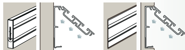
Aufputzmontage
