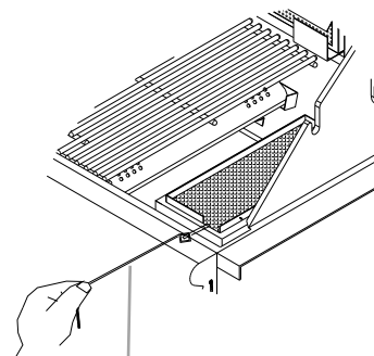
A A. Porte-allumette
