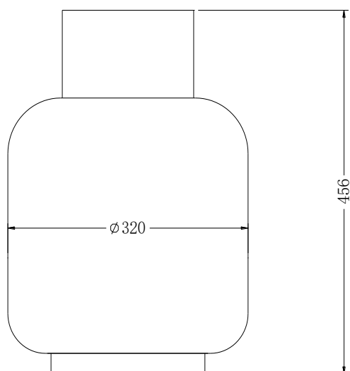
Réservoir de propane : hauteur = 456mm , diamètre = 320mm
