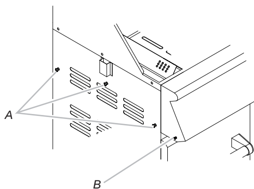
A. Vis du panneau latéral du gril
