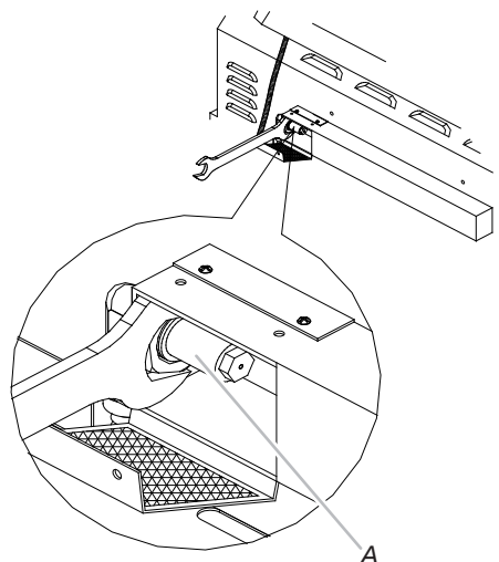
A. Tuerca del orificio
