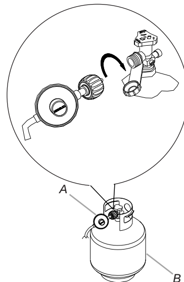
A. Ensamblaje de regulador de presión/manguera de gas
