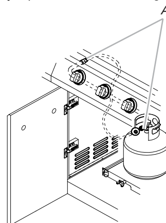
A. Ensemble détendeur/tuyau
