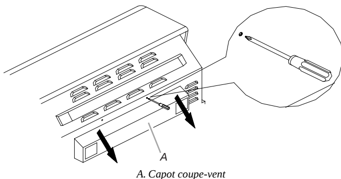
A. Capot coupe-vent
