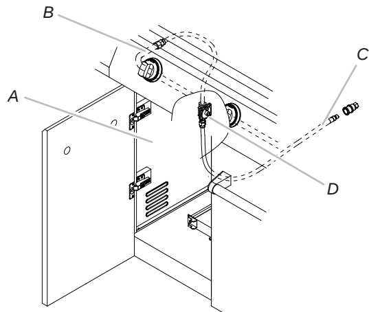
A. Panneau de gauche B. Tubulure de distribution C. Tuyau à gaz en PVC de 10 pi. (3,0 m) D. Ensemble détendeur/tuyau pour gaz naturel
