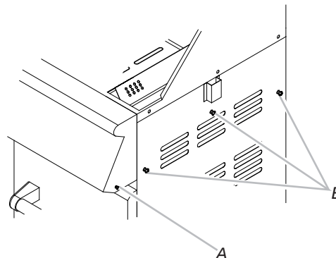
A. Tornillo del panel de control del asador
