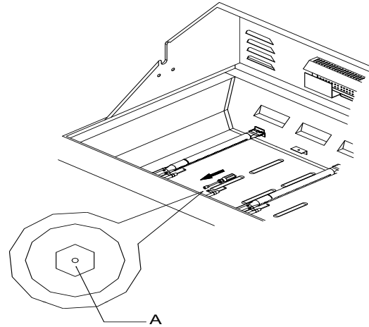
A. Orificio del quemador principal
