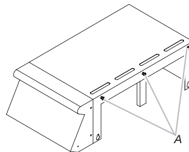
A. Tornillos del estante lateral
