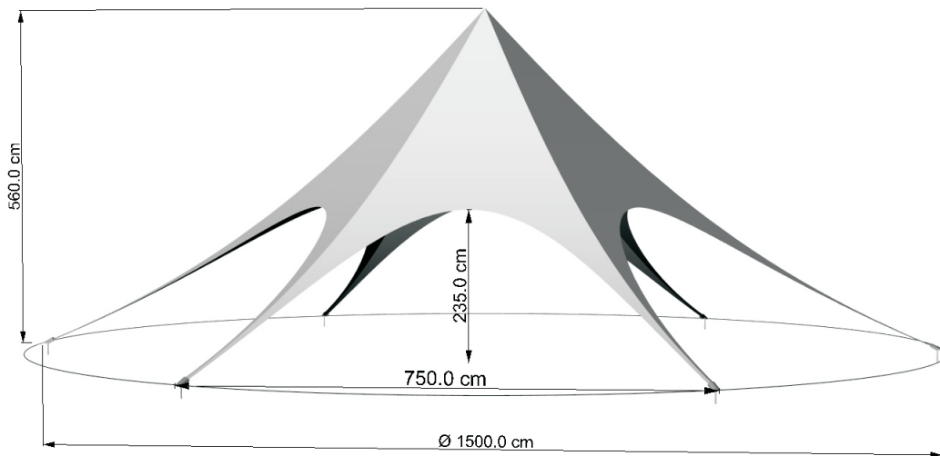
TPSP 150 - 6 fins
