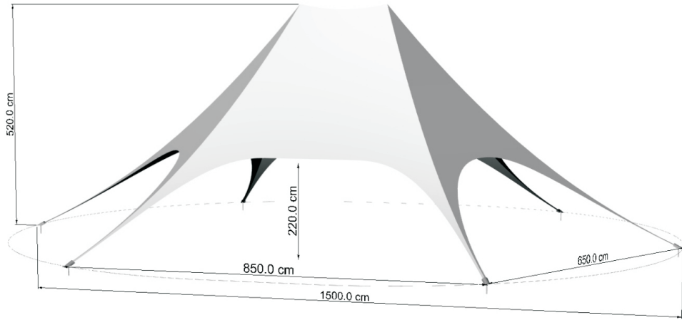
TPDP 150 - 6 fins
