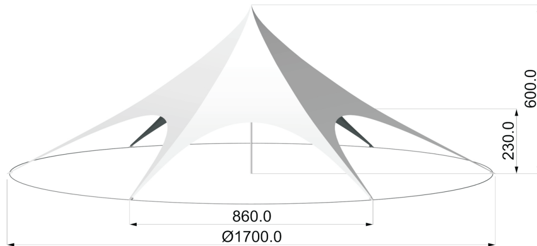
TPSP 170 - 6 fins
