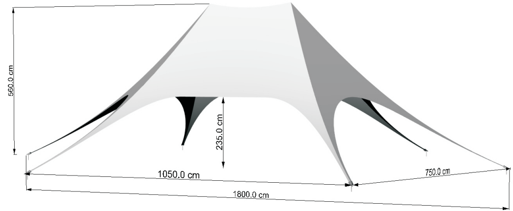
TPDP 180 - 6 fins
