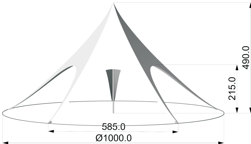
TPSP 100 - 5 fins
