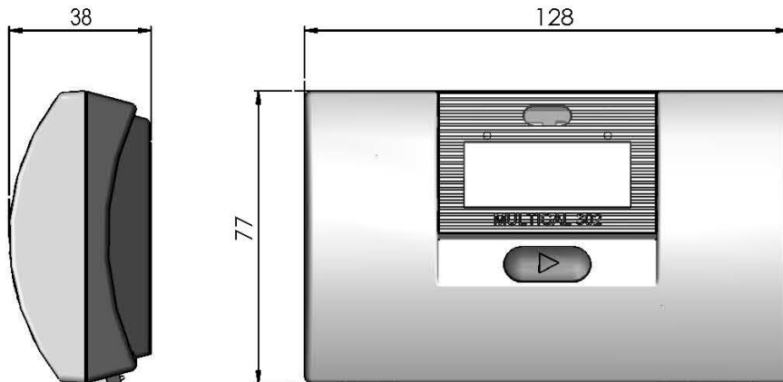
Wandmontiertes Rechenwerk
