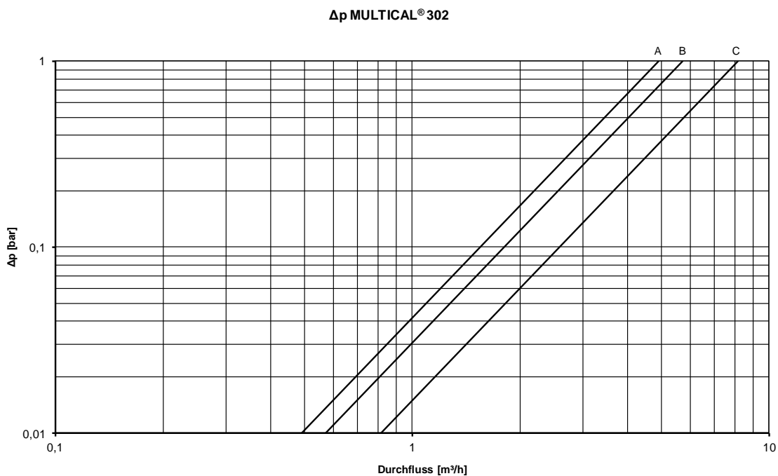
Diagramm 2: Druckverlustkurven
