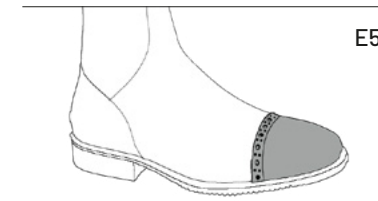
E5 Punched holes over the toe cap Vorschuhkappe mit Lochmusternaht Bout avec trous
