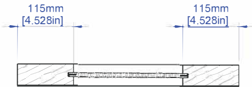
SECTION B-B SCALE 1 : 8
