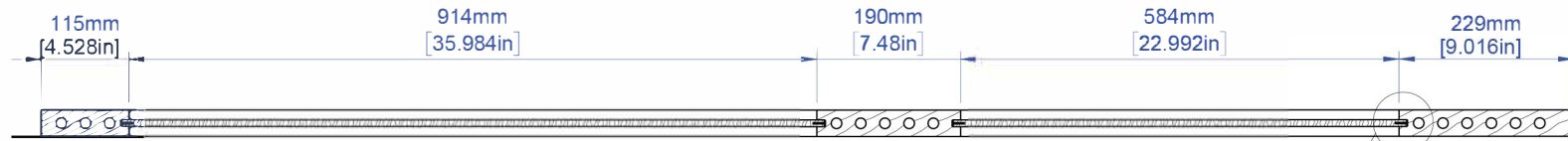
SECTION A-A
