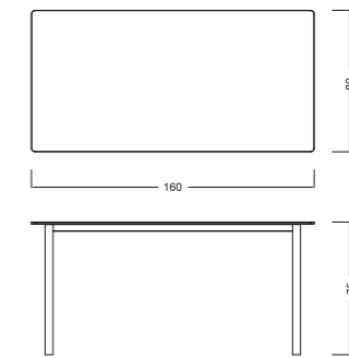
④ TB-11-80160KBT Size: L160×W80×H75cm
