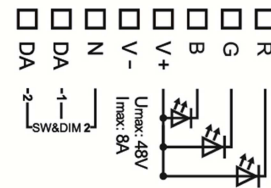
Anschlussplan Dose
