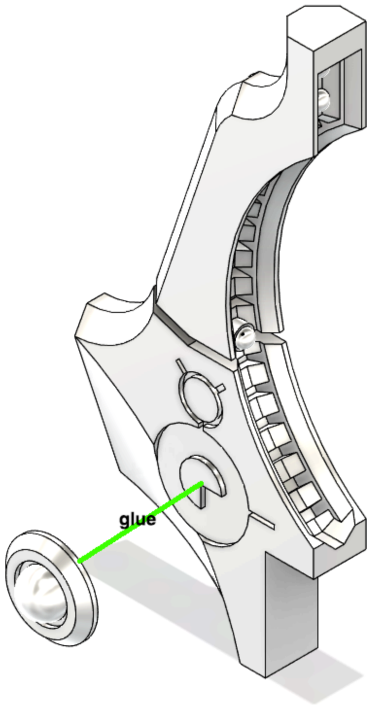
FIN 2 ASSEMBLY
