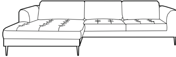
LHF CHAISE SOFA H80 W280 D168CM
