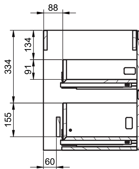
B-B (1 : 10)
