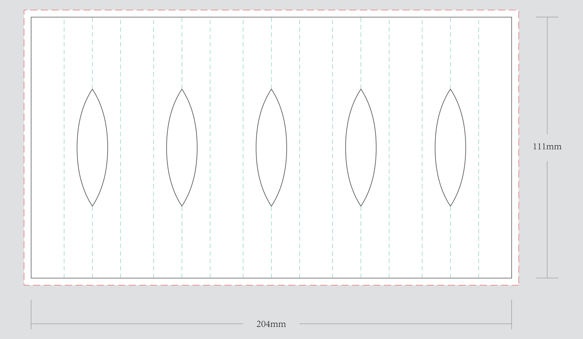
210g单铜纸 注：内托所有的虚线做针孔线 内托一定要贴在盒里
