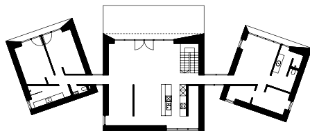
PIRMO AUKŠTO PLANAS
