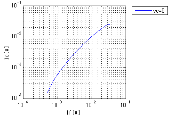
IcTemp[If]
