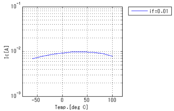
IcTemp[If]
