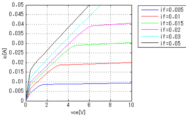
IcIf[Vce]
