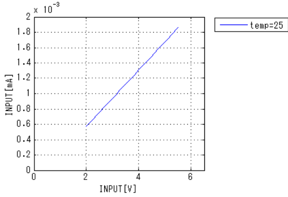
IN_VIN[Temp]
