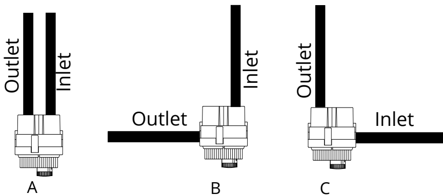
Fig. 3 Plumbing options
