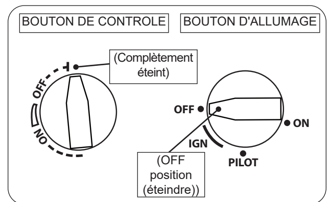
Fig. 73-2 Arrêt manuel
