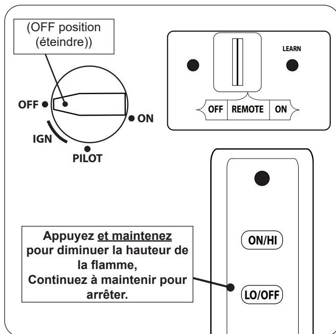
Fig. 74-2 Arrêt à distance
