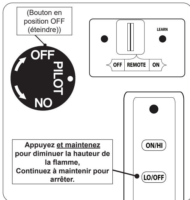
Fig. 77-2 Arrêt à distance
