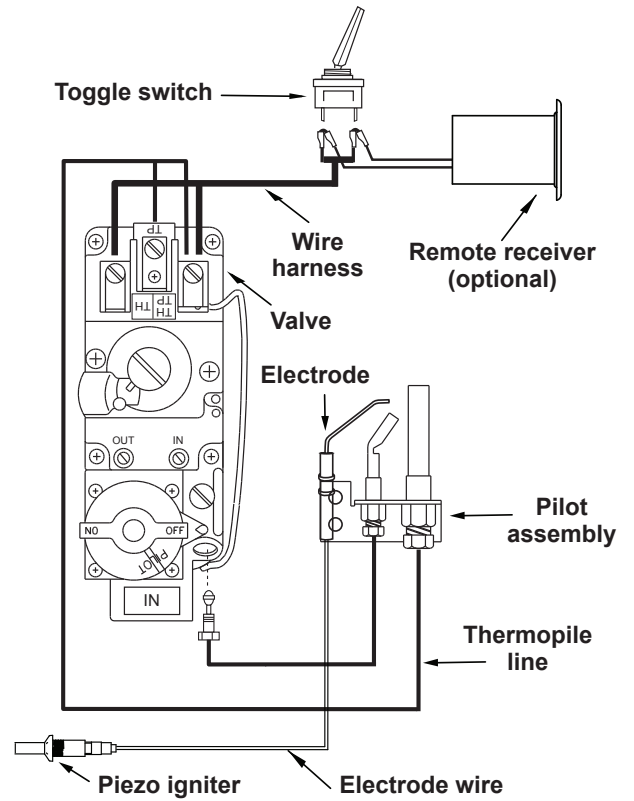
Fig. 59-2
