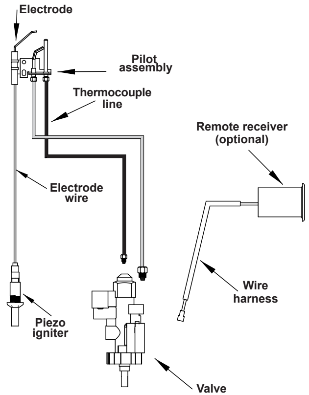
Fig. 59-4
