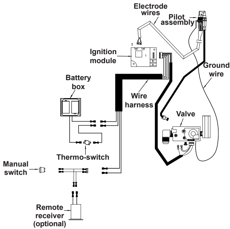
Fig. 59-1
