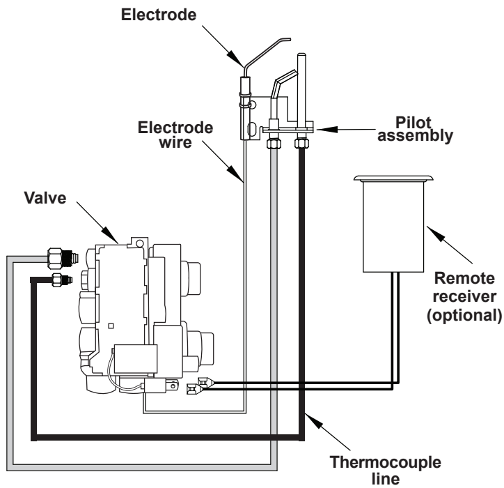
Fig. 59-3
